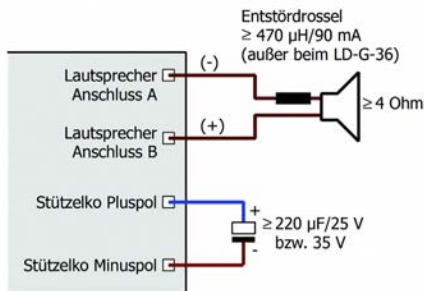
Fig. 4: Anschluss eines Stützkelkos zur Verbesserung der Spannungsversorgung und einer Entstördrossel am Lautsprecher
